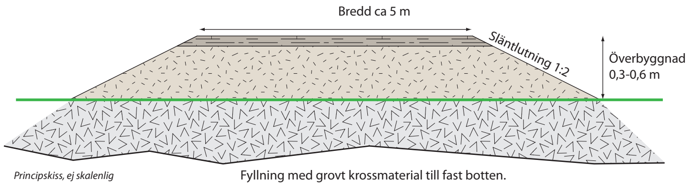
Typsektion 2, torvmark
