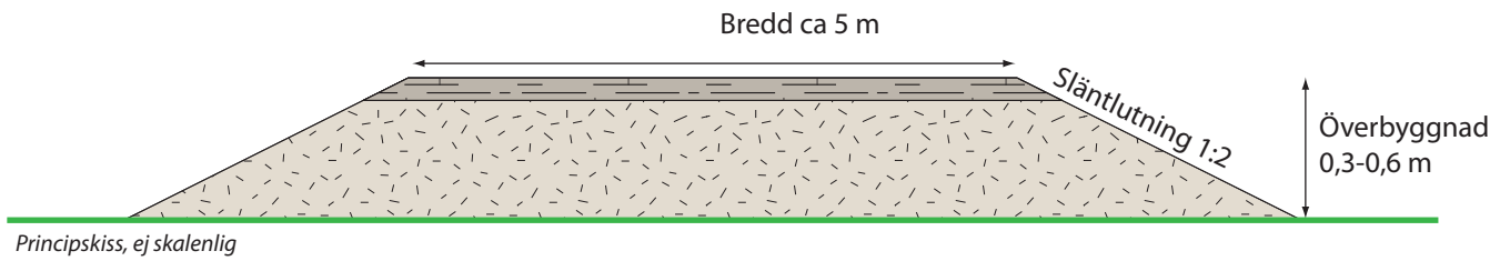
Typsektion 1, moränmark
